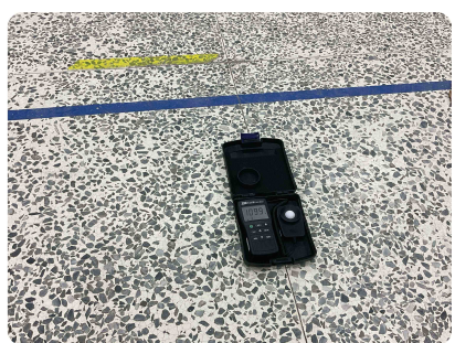
調光使用100%，照度 1099
